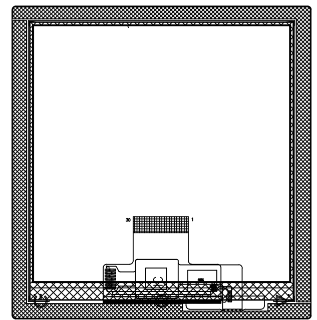
TPM 出货示意图 FPC焊接后翻折固定
