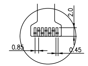
A: TP金手指焊接区域 缩放比例2:1
